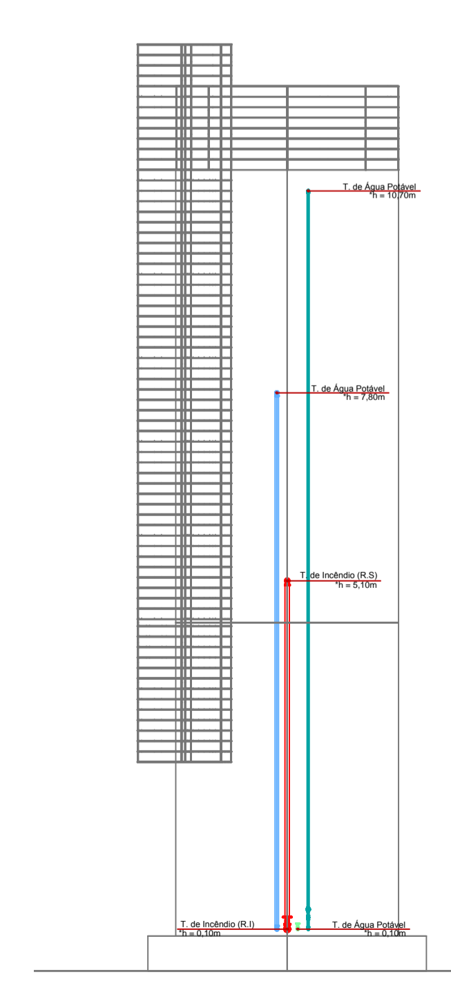
VISTA NORTE - ALTURA DAS SAÍDAS ESC.:1/75
