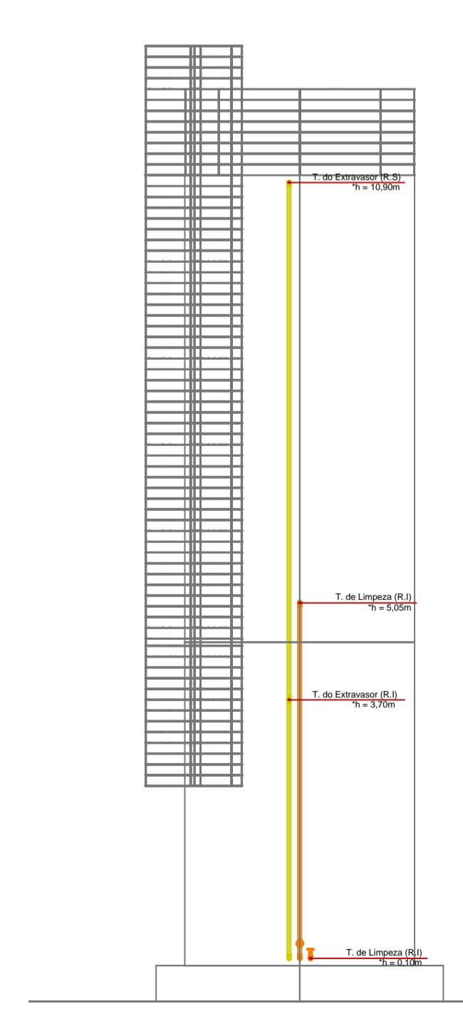
VISTA LESTE - ALTURA DAS SAÍDAS ESC.:1/75
