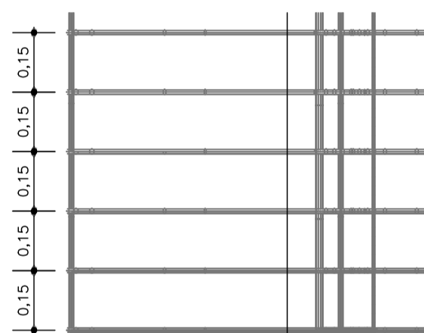
PLANTA BAIXA - IMPLANTAÇÃO ESC.:1/50
