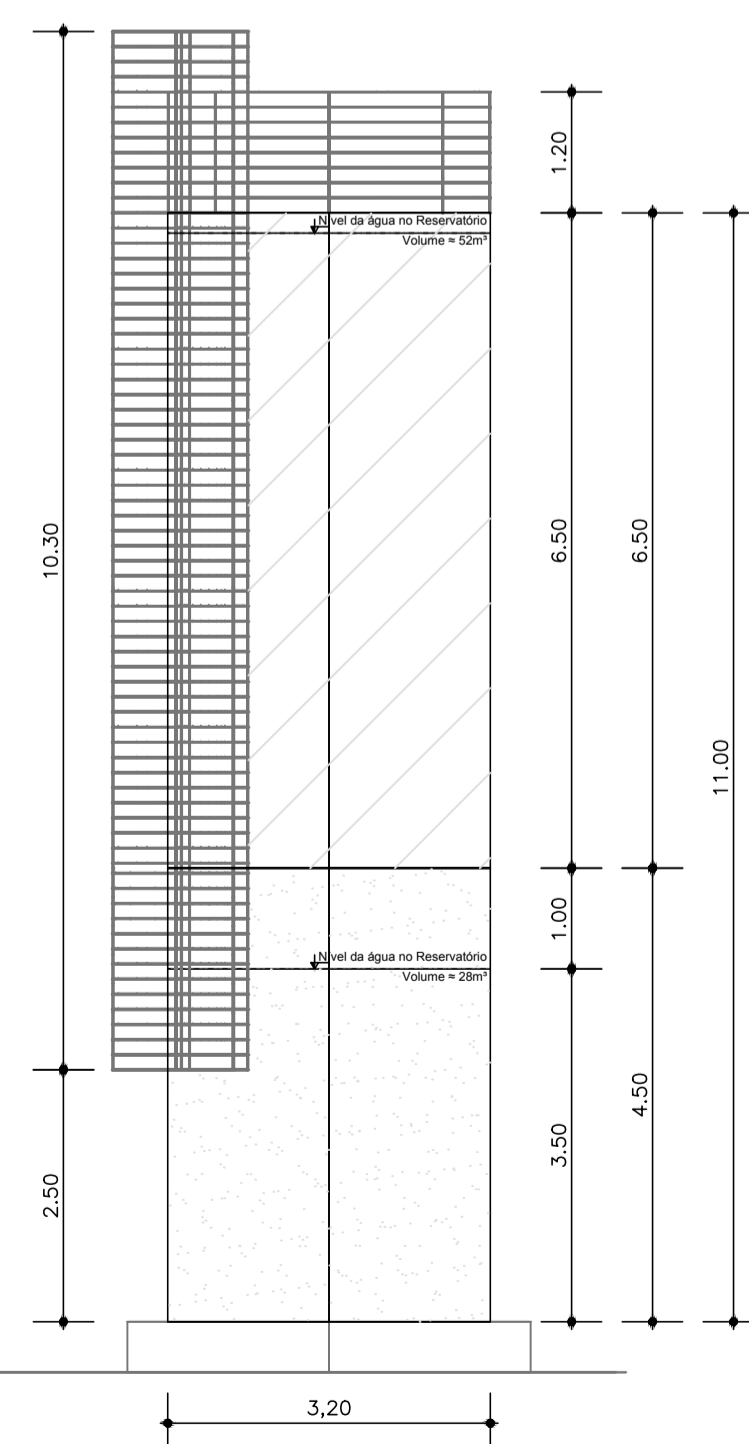
VISTA OESTE - RESERVATÓRIO METÁLICO ESC.:1/75
