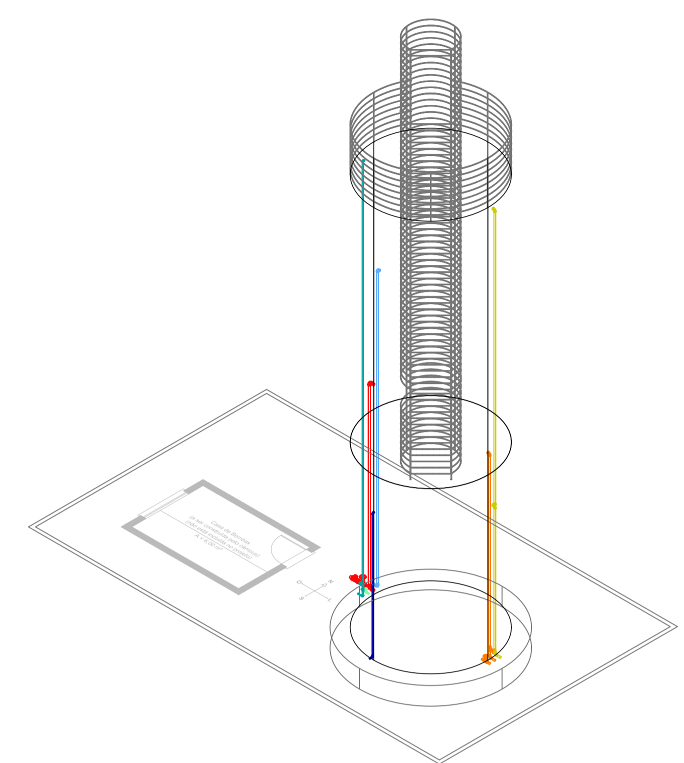
ESTEREOGRAMA - VISTA LESTE ESC.:1/75
