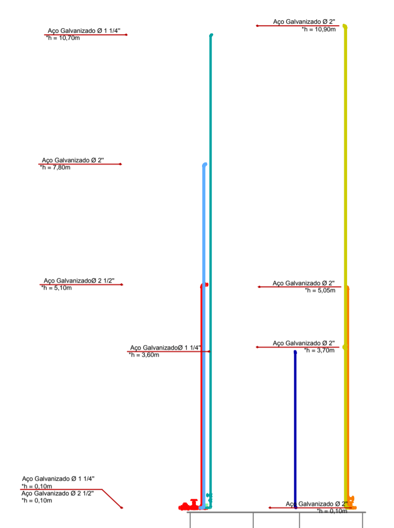
ESQUEMA DAS TUBULAÇÕES ESC.:1/75
